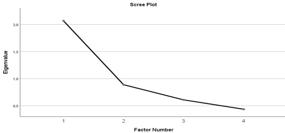
Şekil 2. İkinci Düzey AFA Yamaç-Birikinti Grafiği
