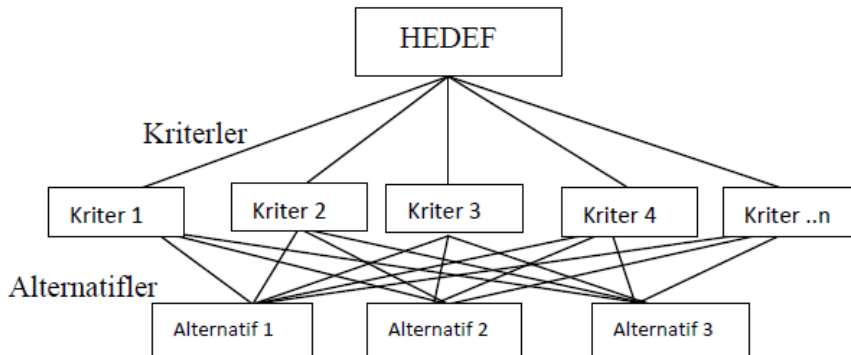
Şekil 3. AHP Yönteminin Hiyerarşik Yapısı
